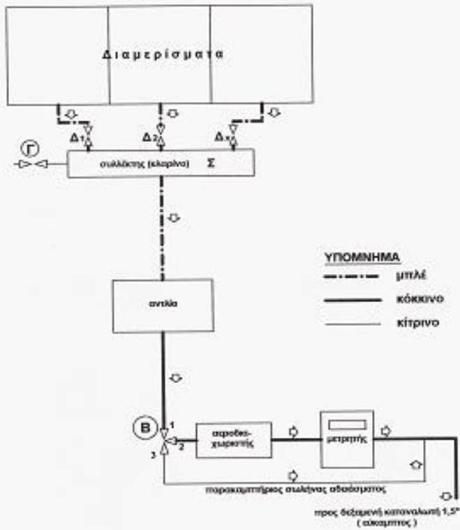
ΚΥΚΛΩΜΑ ΚΑΥΣΙΜΟΥ ΣΕ ΒΥΤΙΟΦΟΡΑ ΠΕΤΡΕΛΑΙΟΥ ΘΕΡΜΑΝΣΗΣ (χωρίς σύστημα αναρόφησης)
